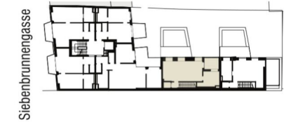
Grundriss 2. Obergeschoss
