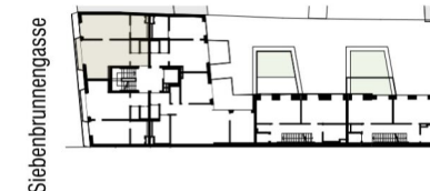
Grundriss 1. Obergeschoss
