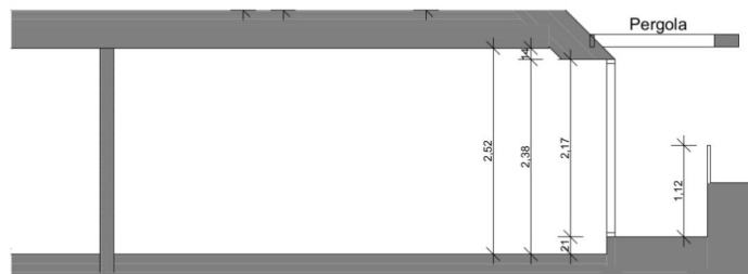
Schnitt 2/64 A
