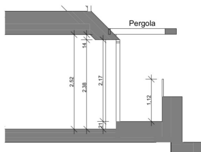
Schnitt 2/65 A
