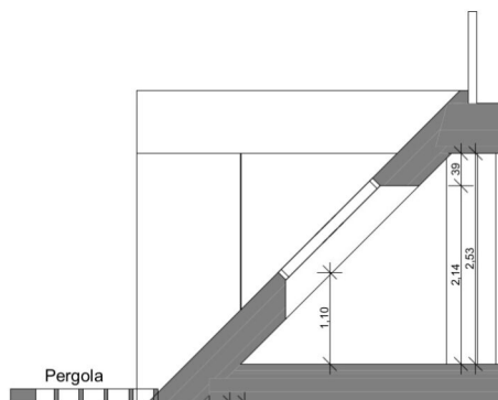
Schnitt 1/77 A
