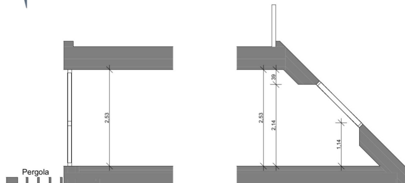
Schnitt 2/70 A
