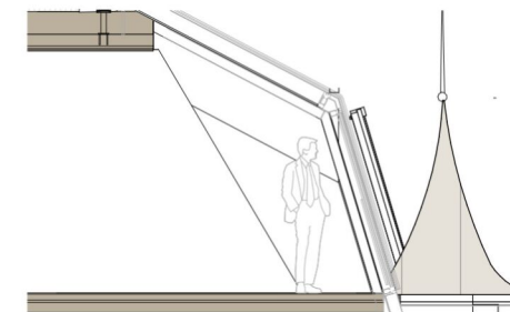
SCHNITT TOP25
