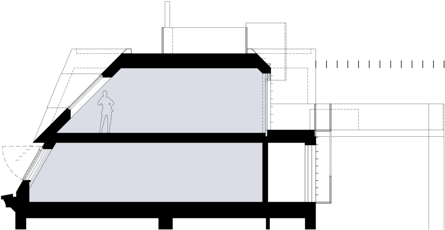
SNITT
