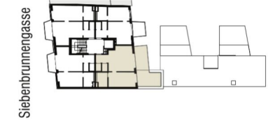
Grundriss 4. Obergeschoss
