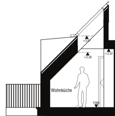
Schnitt
