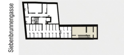
Grundriss Untergeschoss
