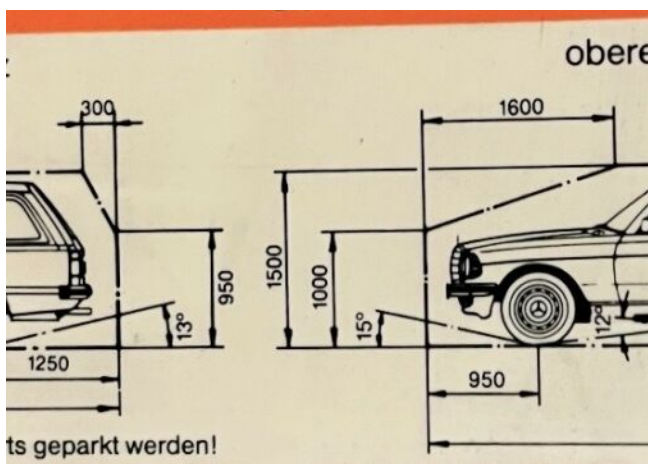
Abmessungen Garage
