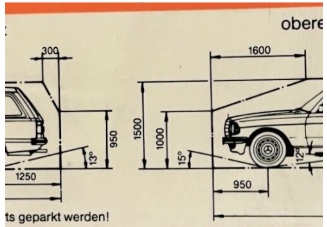
Abmessungen Garage
