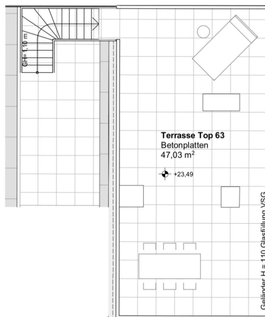
Grundriss Dachterrasse
