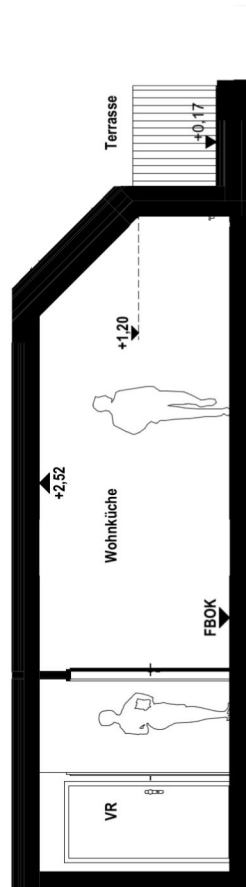
Schnitt
