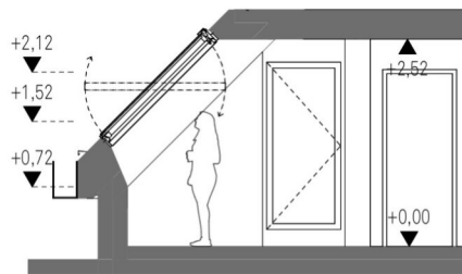
Schnitt 1
