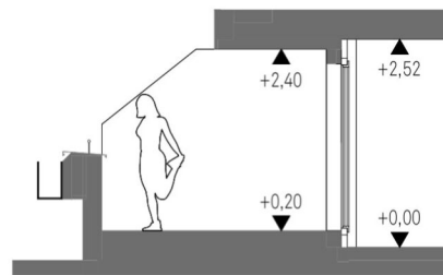
Schnitt 2
