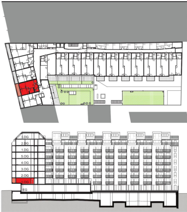
TOP 11 1.OBERGESCHOSS 2 ZIMMER
