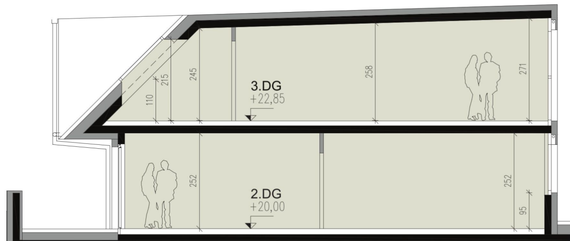
SCHNITT A
