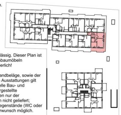
Übersichtsplan 1.OG
