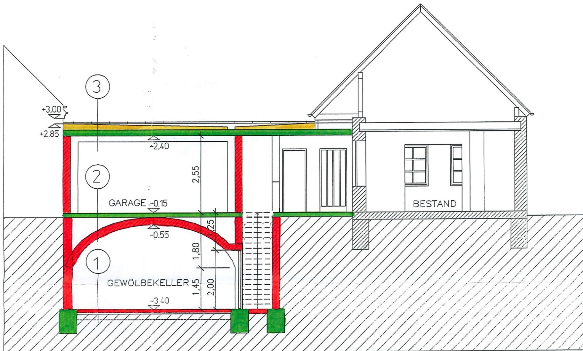
SCHNITT Garage
