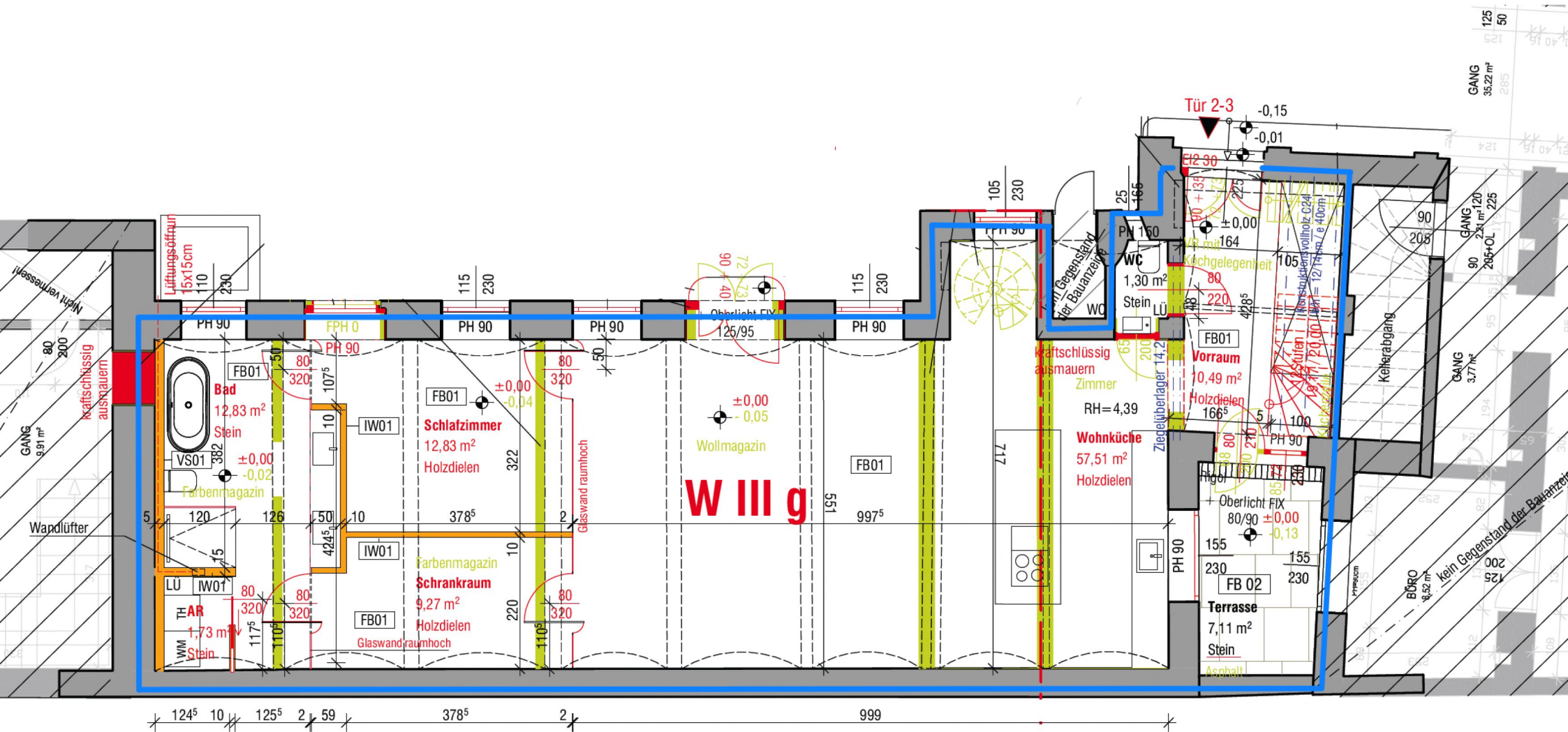
Grundriss EG 1:100
