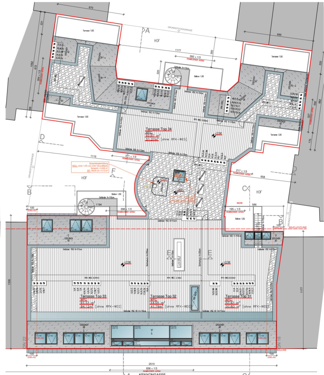
DACHDRAUFSICHT
