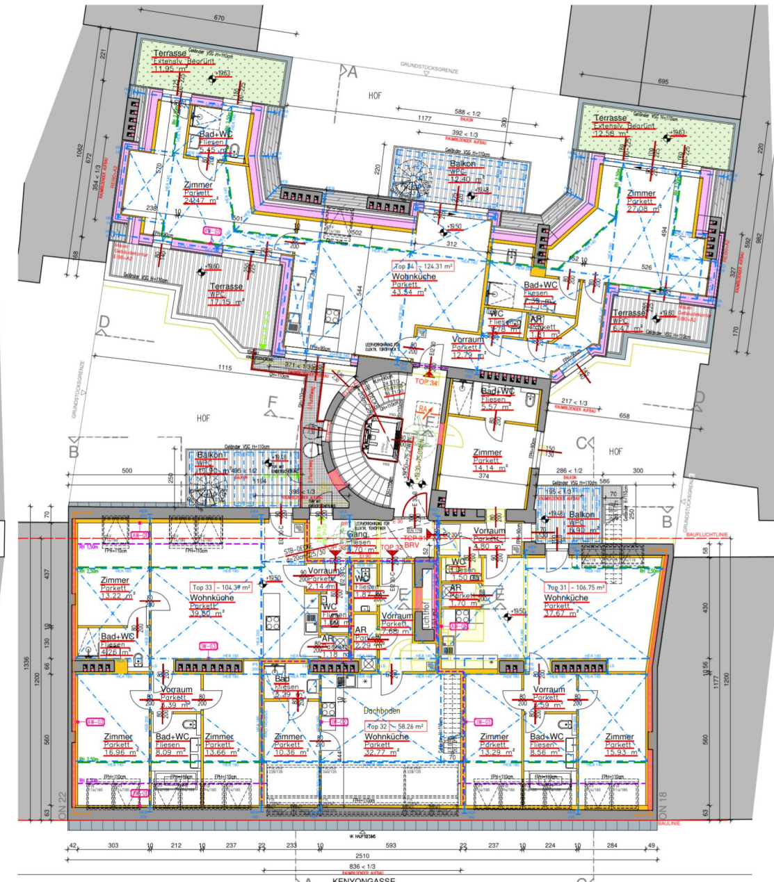
1. DACHGESCHOSS
