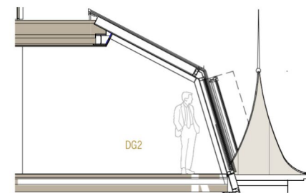
SCHNITT TOP22
