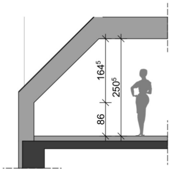
SCHNITT 2-2
