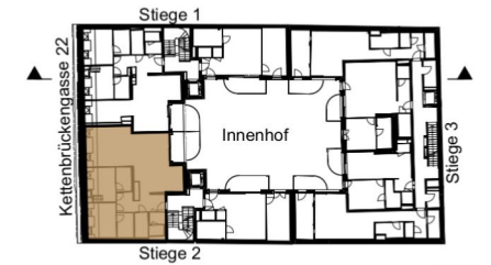
OG3
