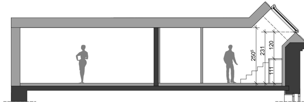
SCHNITT 3-3
