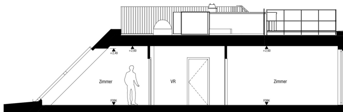
Schnitt
