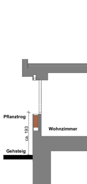
Fassadenschnitt
