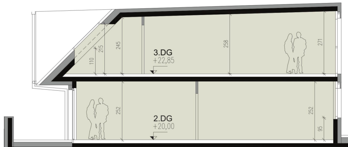
SCHNITT A
