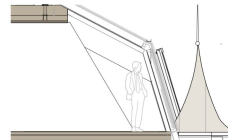
SCHNITT TOP25
