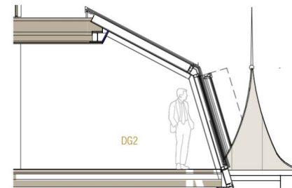
SCHNITT TOP22
