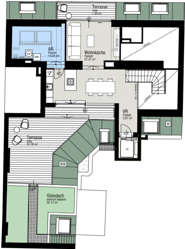
2. DACHGESCHOSS Maßstab 1:200
