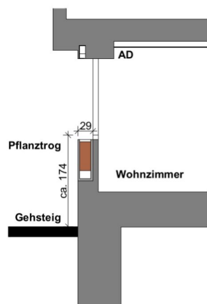
Fassadenschnitt
