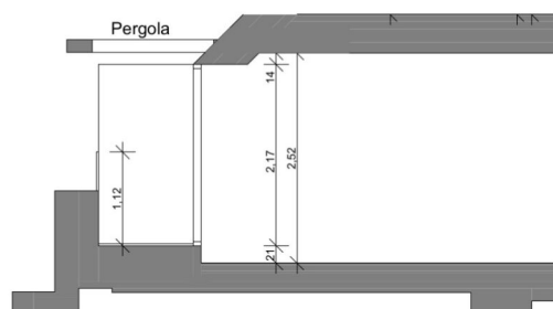
Schnitt 1/73 A
