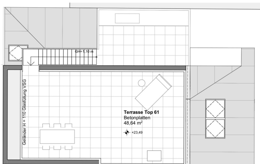
Grundriss Dachterrasse
