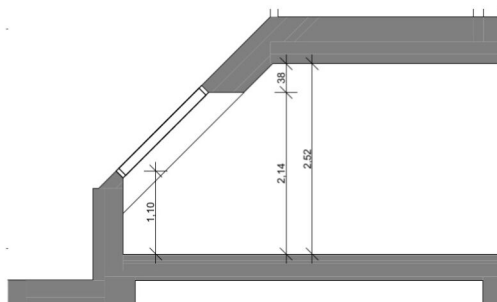
Schnitt 2/61 A
