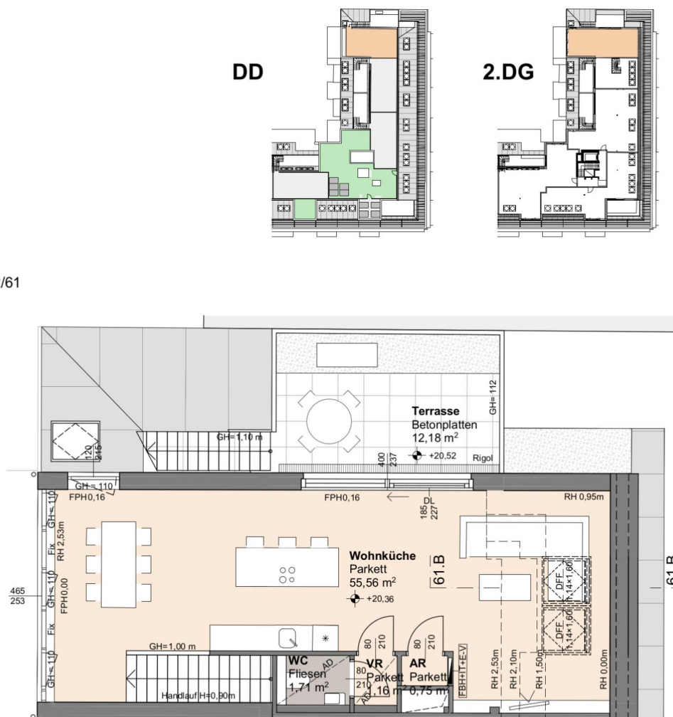
Grundriss 2.Dachgeschoss
