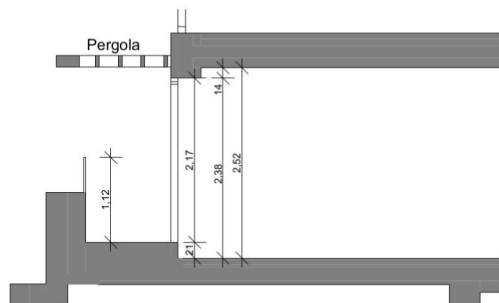
Schnitt 2/67 A
