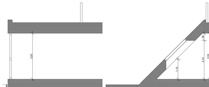
Schnitt 1/78 B
