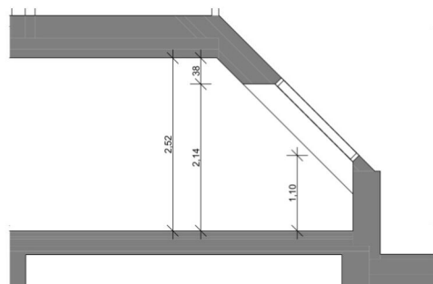
Schnitt 1/76 A
