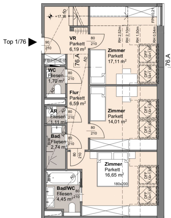
Grundriss 1.Dachgeschoss
