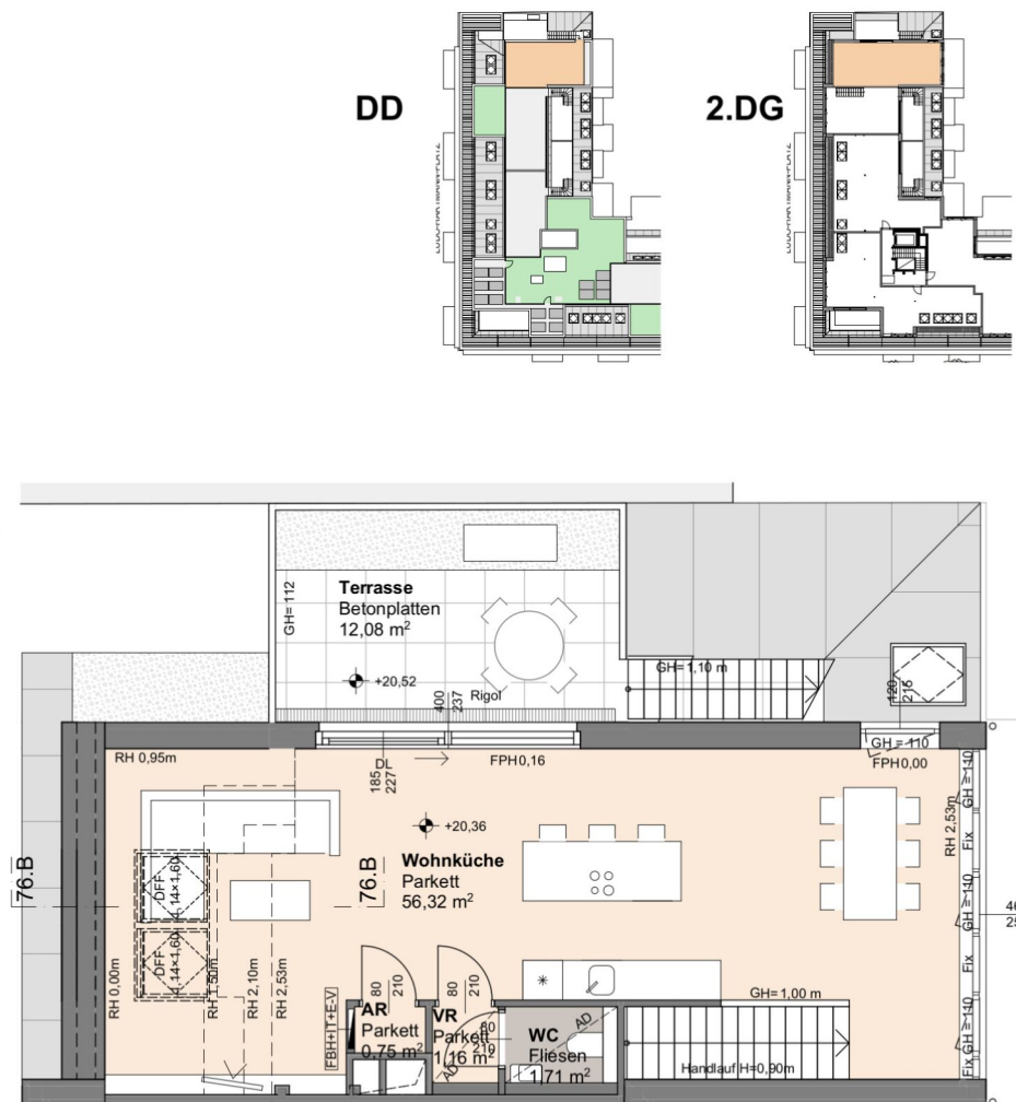
Grundriss 2.Dachgeschoss
