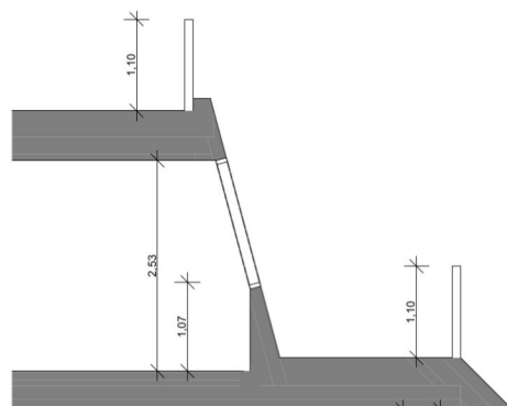
Schnitt 1/77 B
