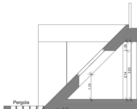
Schnitt 1/77 A
