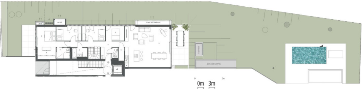
ERDGESCHOSS groundfloor
