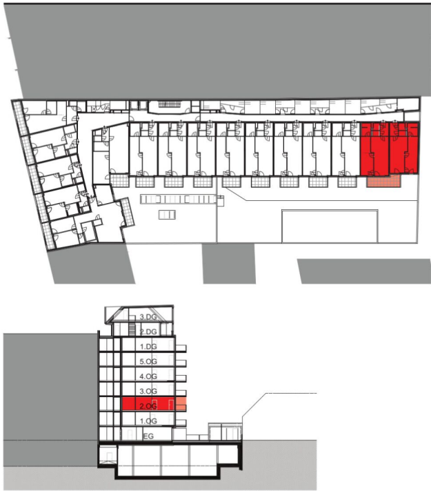
TOP 38+39 - Variante 1 2.OBERGESCHOSS 4 ZIMMER
