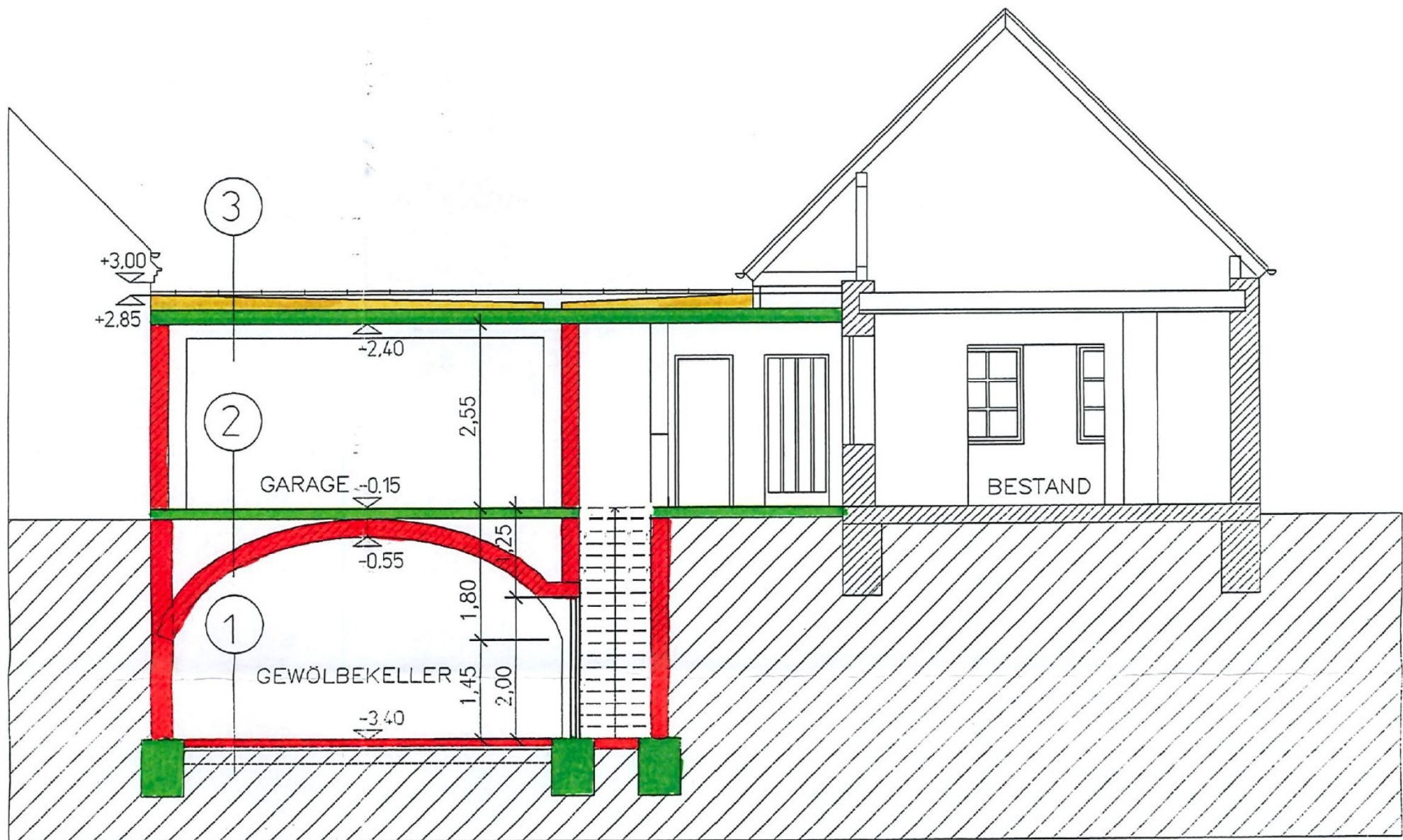
SCHNITT Garage
