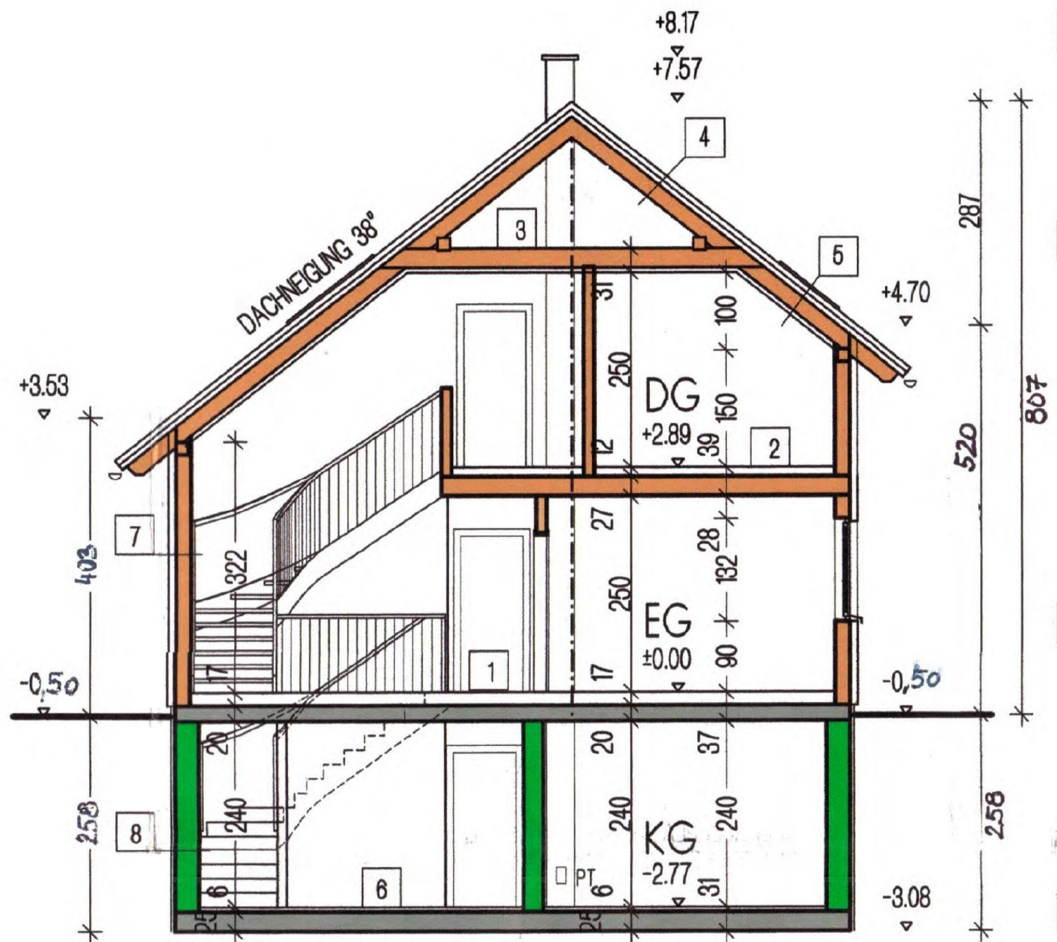
SCHNITT A-A
